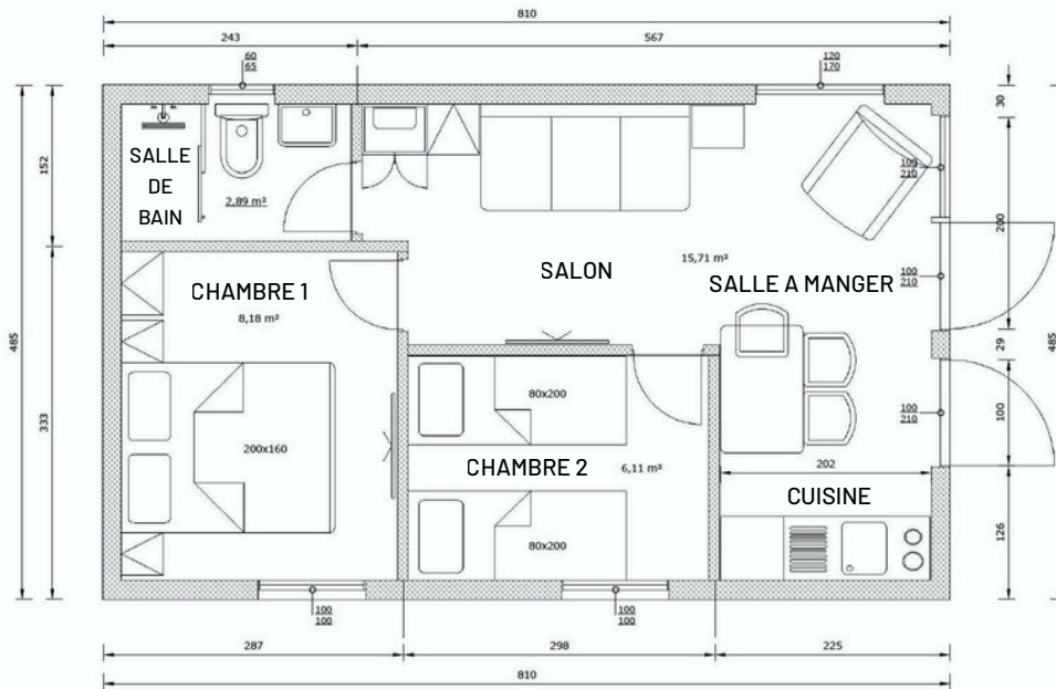
Plan d'étage du mobil-home Louison 40 Comfort
