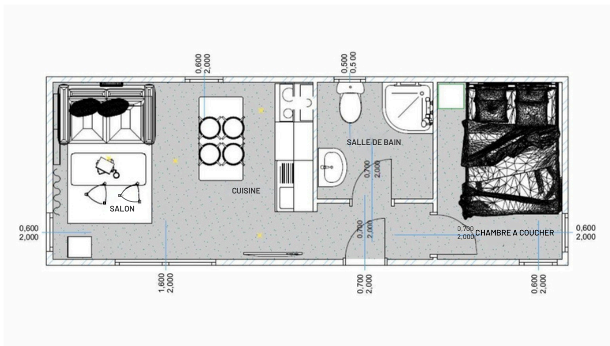
Plan du mobil-home Eden 24
