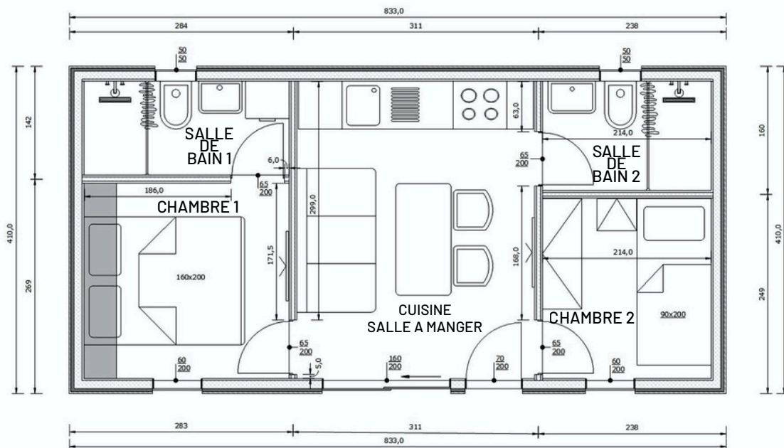
Plan du mobil-home Noa 35
