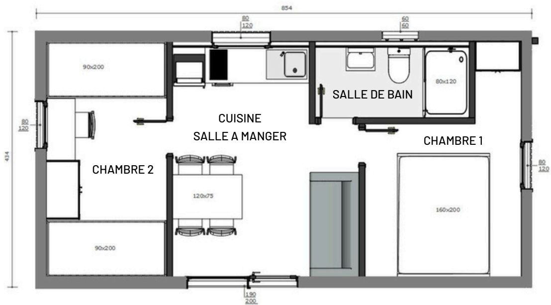
Plan du mobil-home Thaïs 36
