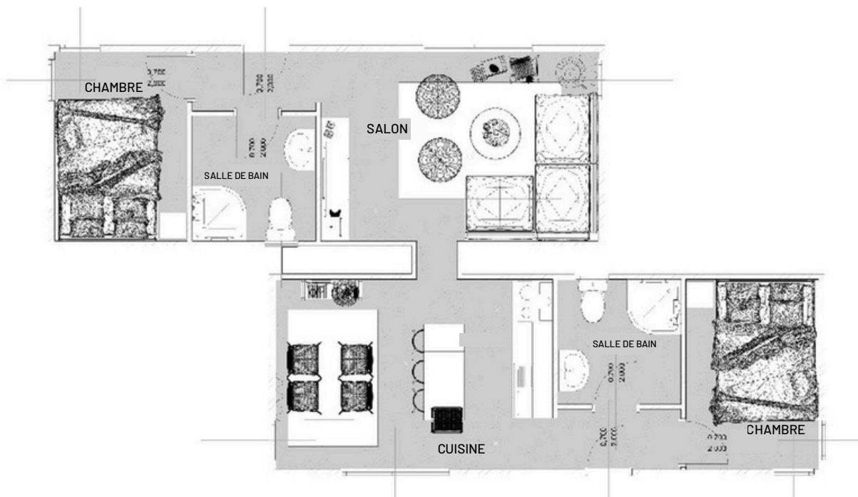
Plan d'étage du mobil-home Léo 48 L ou Z
